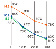
食缶の温度変化
