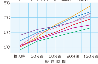
ステンマイルドボックスS 温度テスト結果
