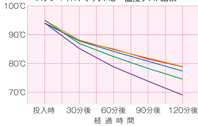
ステンマイルドボックスS 温度テスト結果
